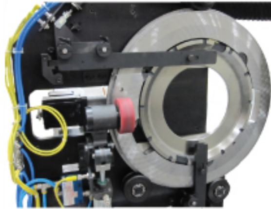
เครื่องเจียรแบบวางรอให้เจียรระโน
